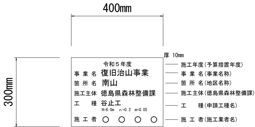
図 1 銘板の寸法及び記載事項
